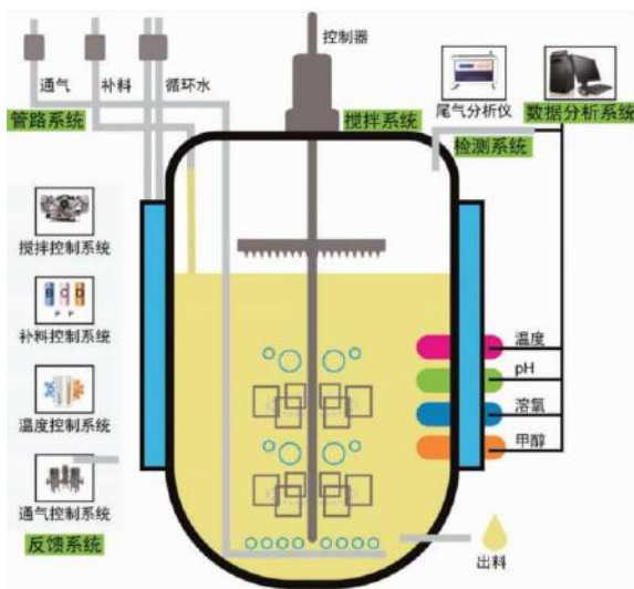
图12 | 经典发酵罐及相关控制参数 (来源: CNKI)
